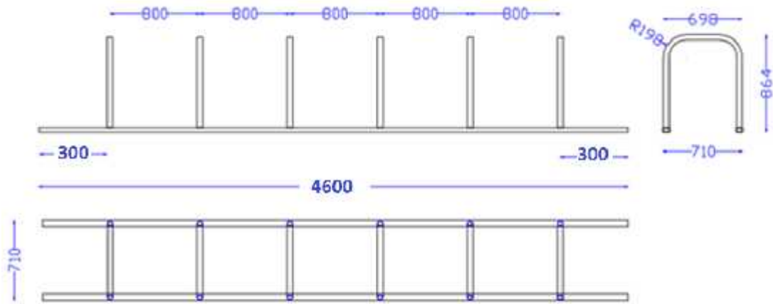
носач бидикла, основа Fe цев 60/40/4, вертикале цеви "fi" φ 48 mm
