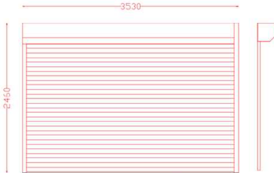
Al роло врата са мотором, бела, ком 2 са кључем споља
